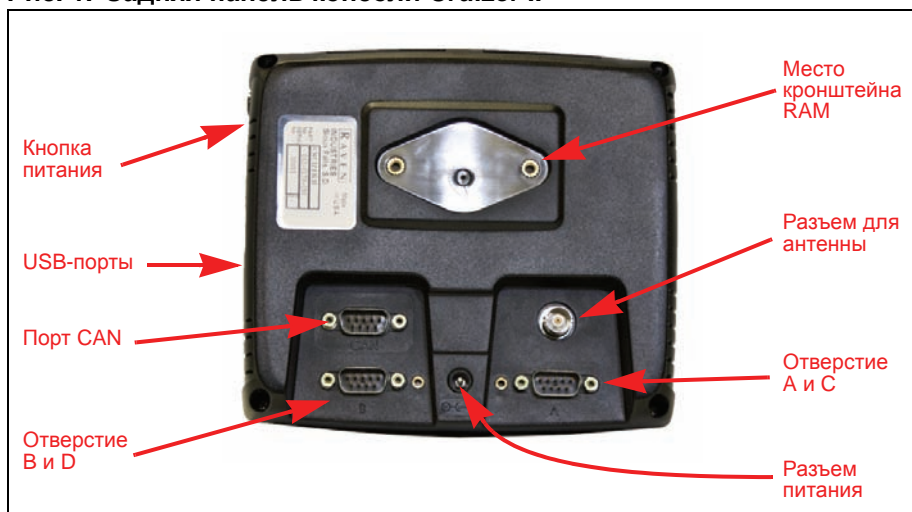
Рис. 1. Задняя панель консоли Cruizer II
